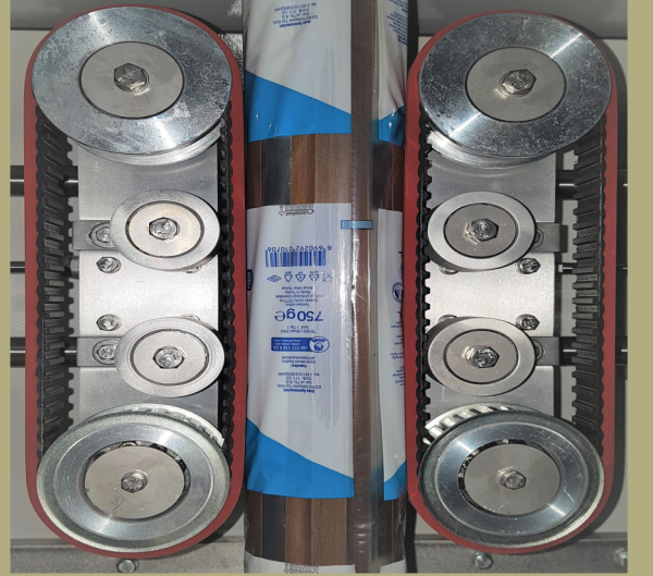
Pnomatik Yanaşmalı Kayışlı Film Çekme Sistemi
